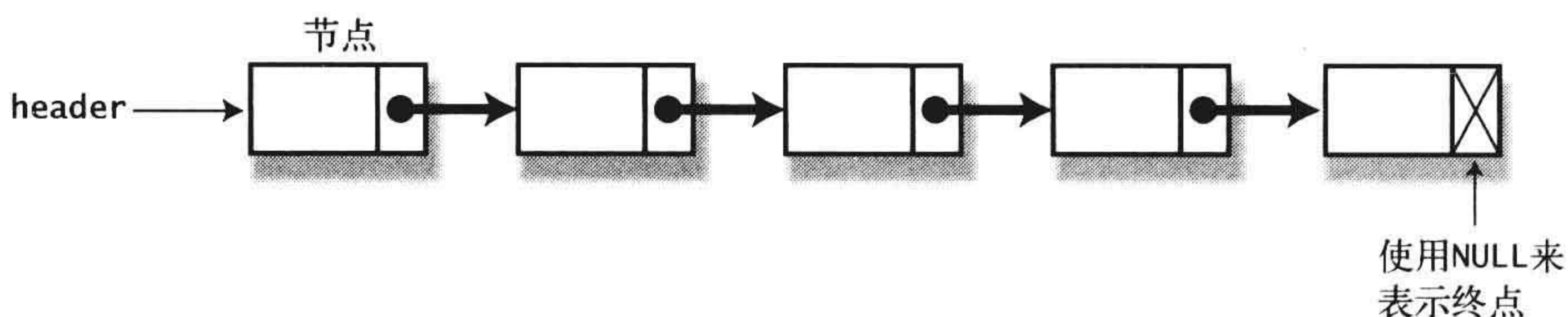
图 5-3 链表
