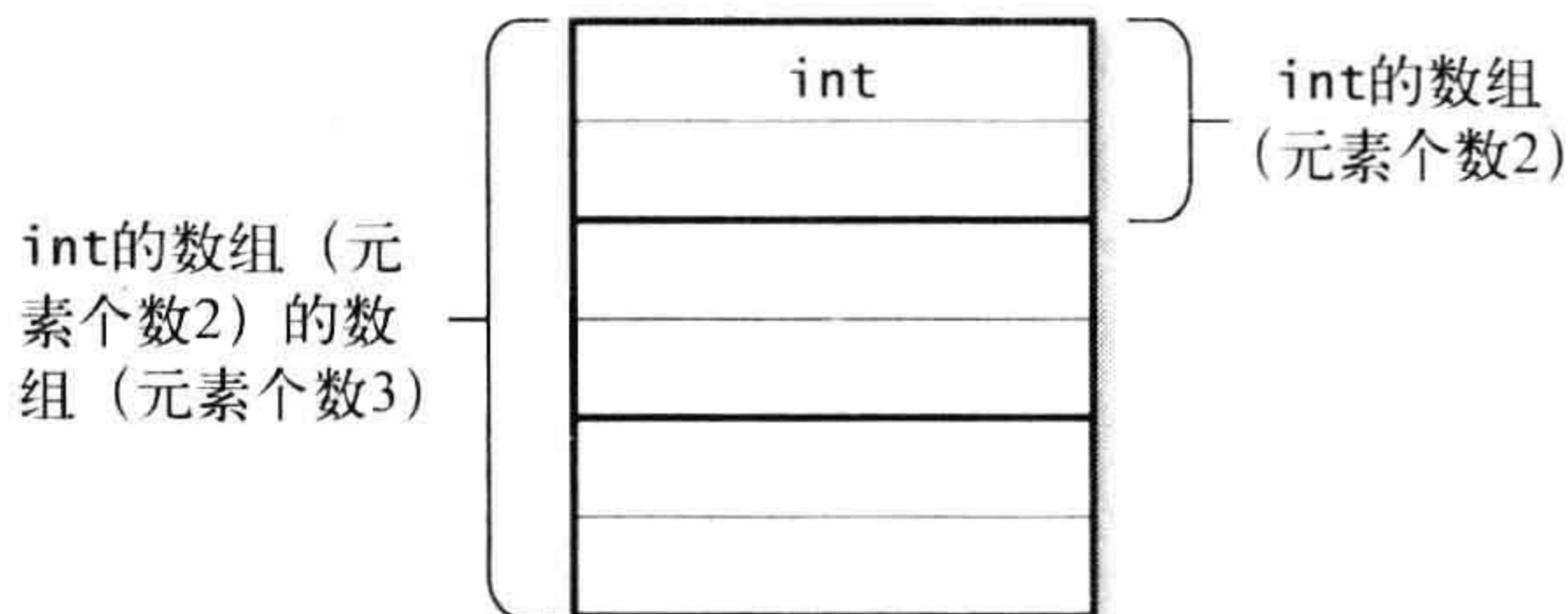
图 3-7 数组的数组
