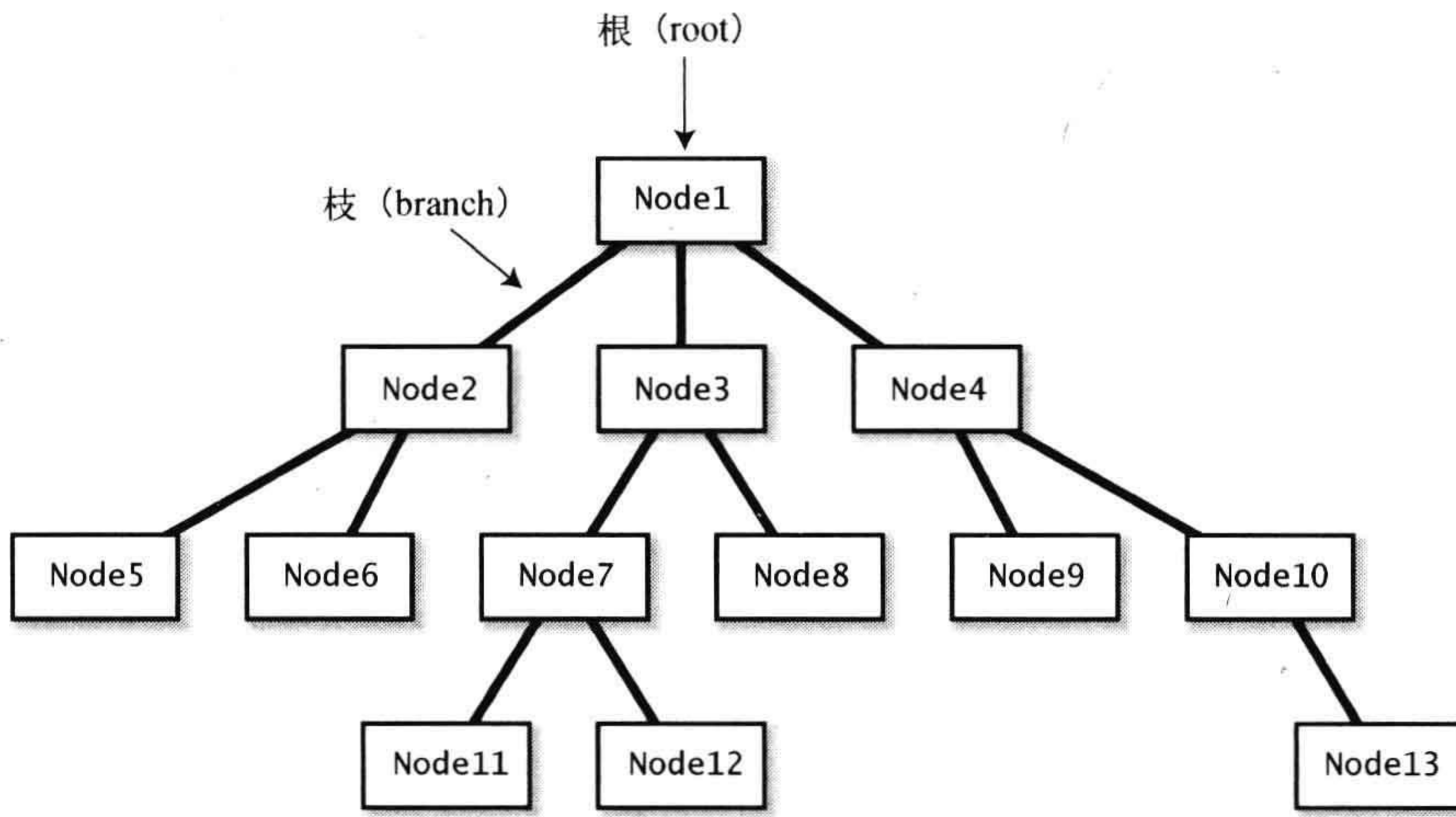
图 5-8 树
