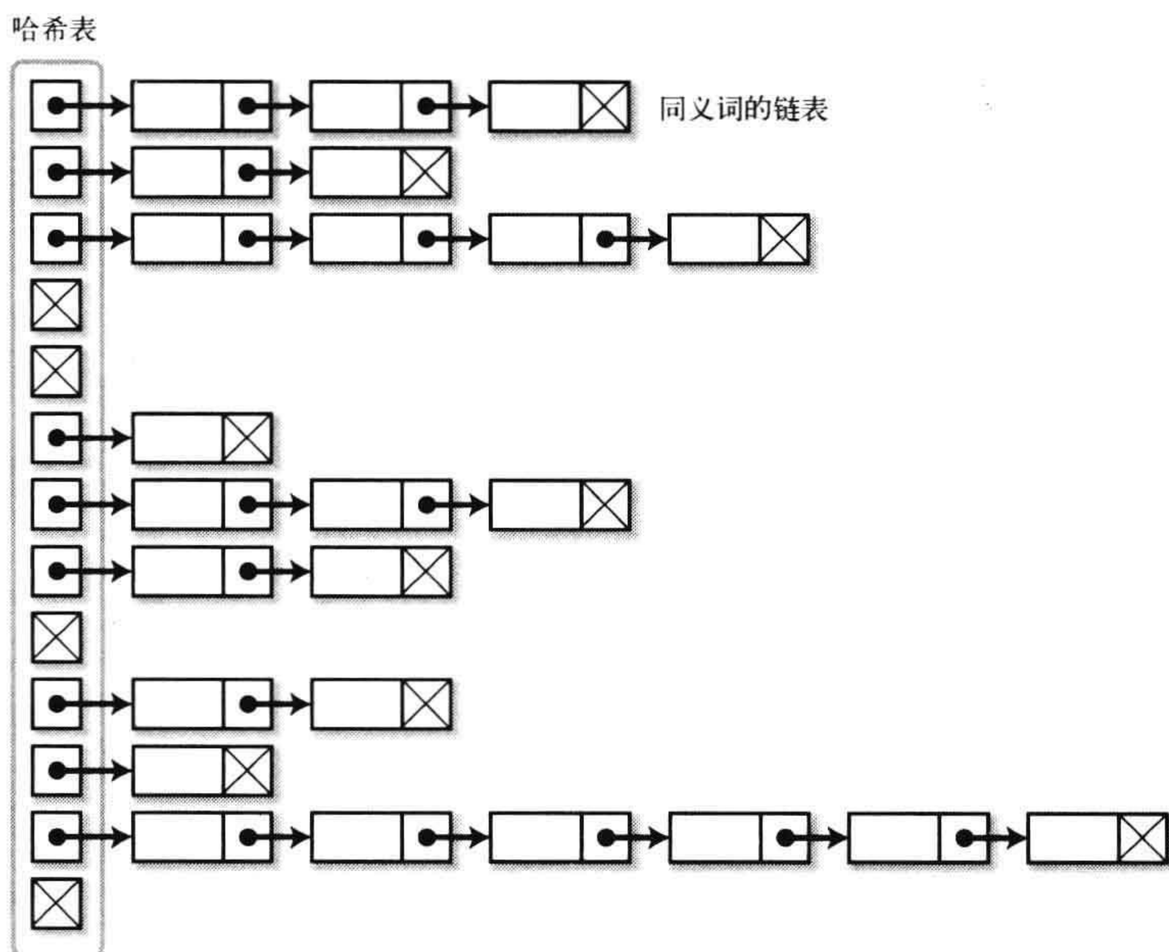
图 5-11 链式哈希
