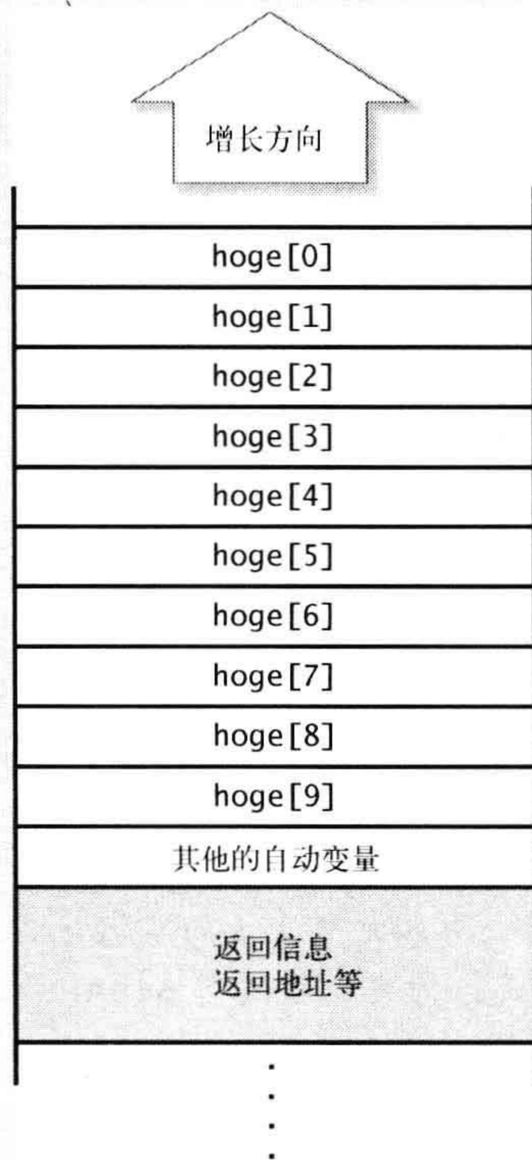
图 2-8 栈中的数组
