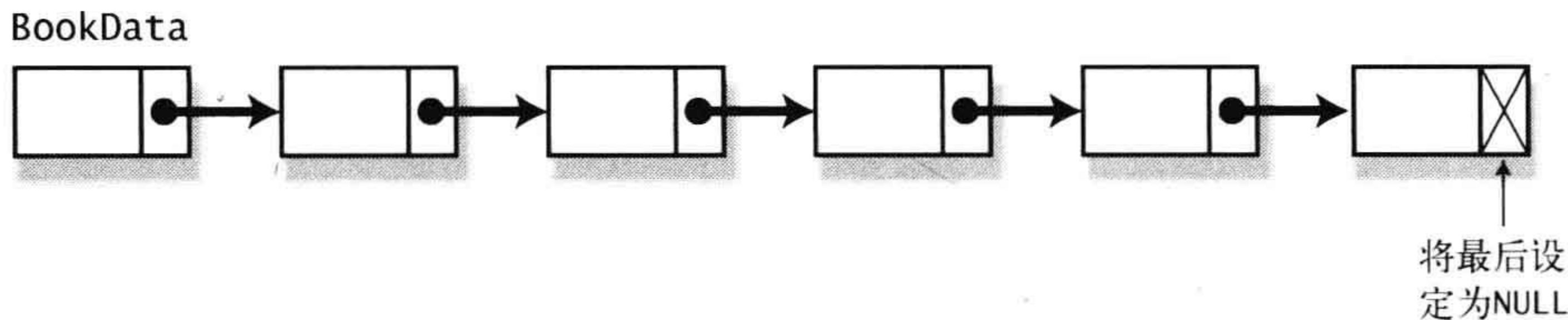
图 2-11 链表
