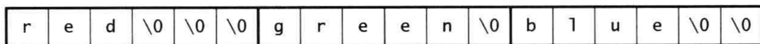
图 3-20 数组的数组
