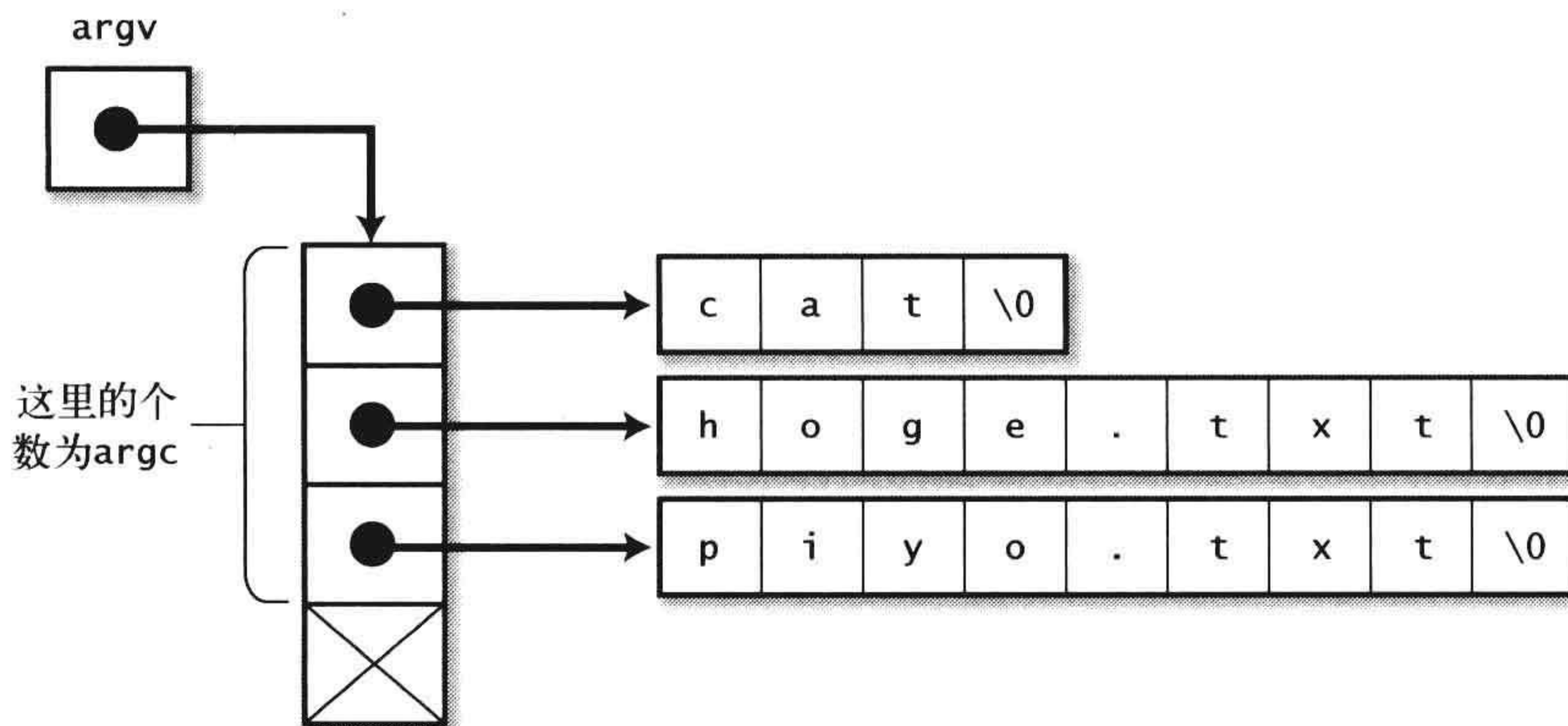
图 4-4 argv 的结构
