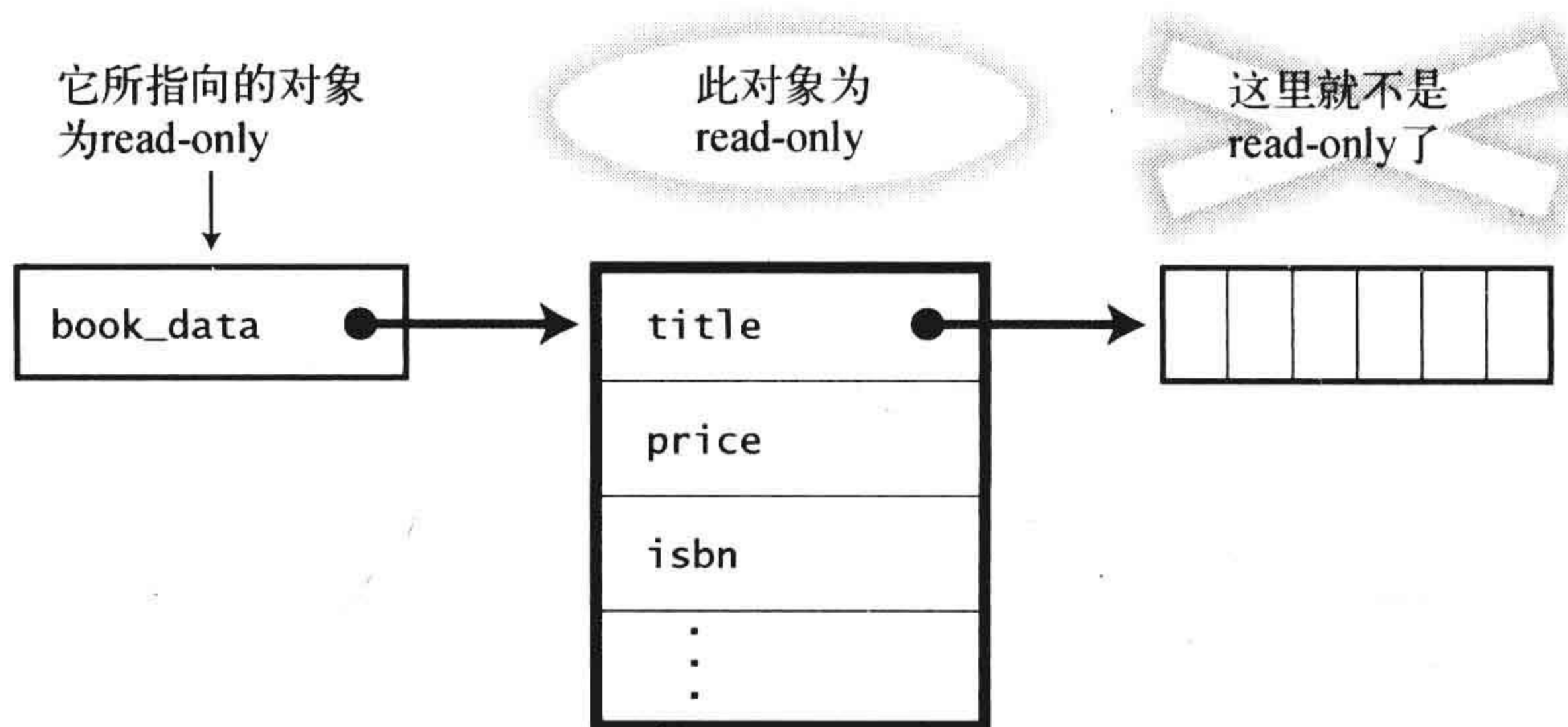
图 3-16 const 的边界
