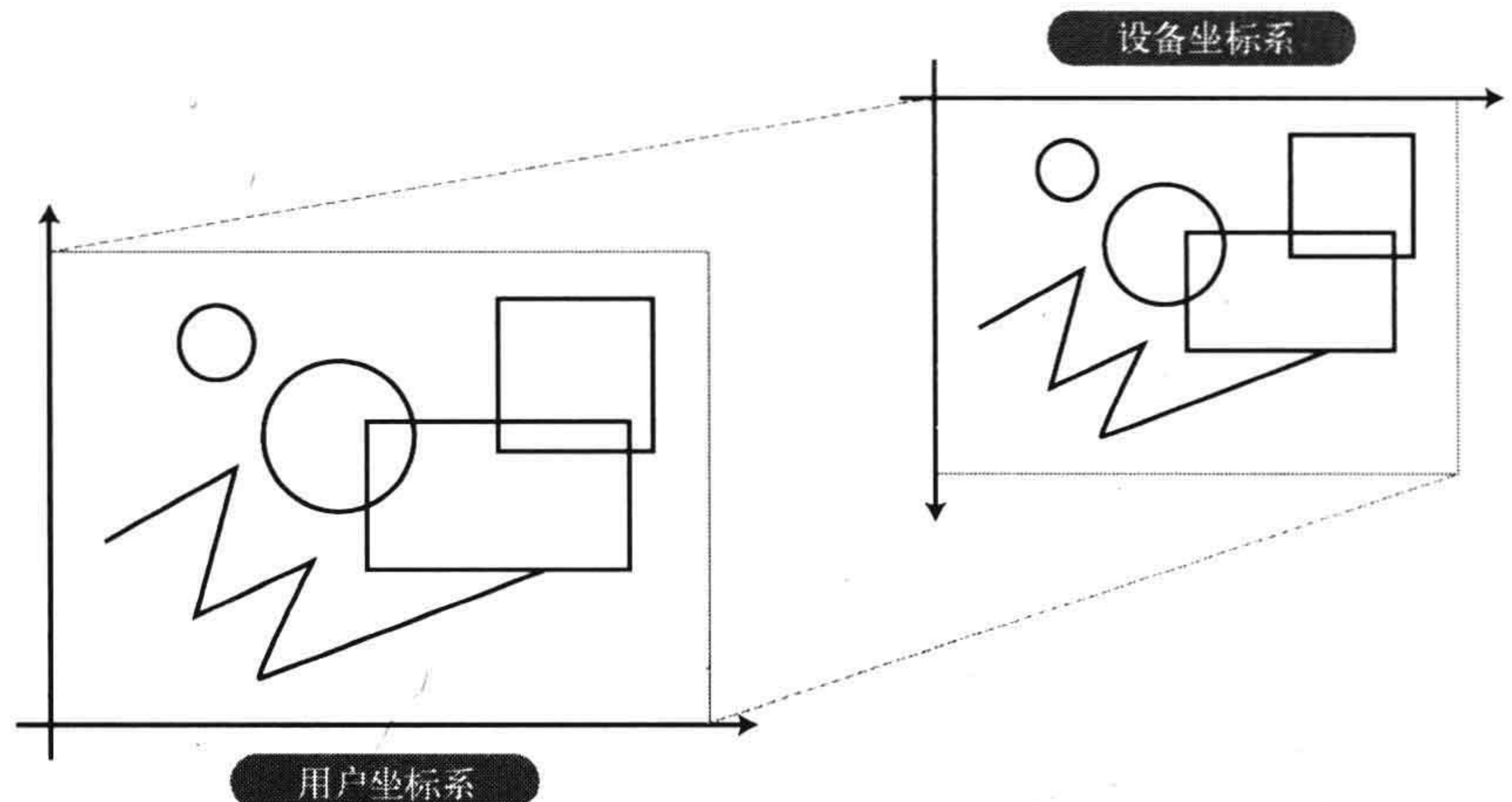
图 5-13 坐标系变换
