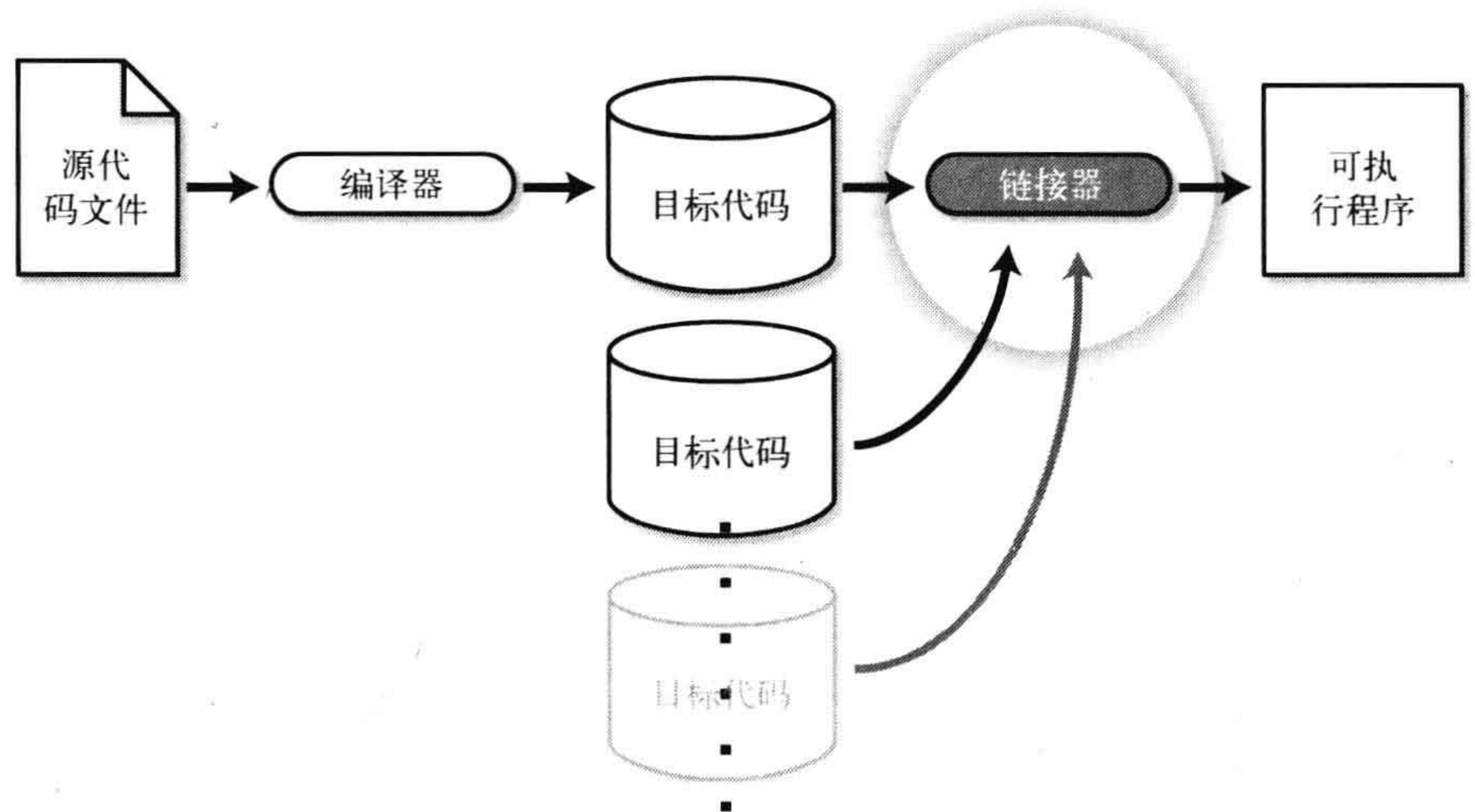
图 2-4 链接器
