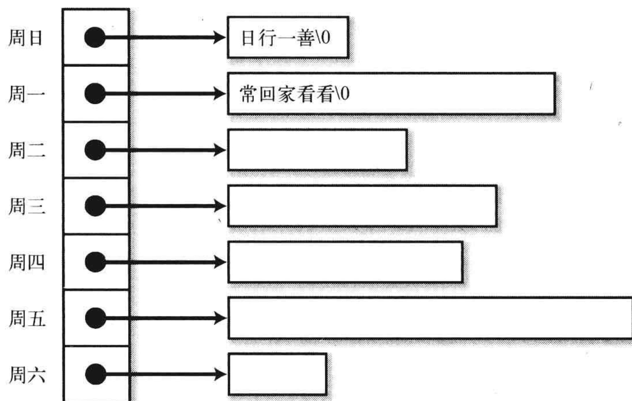
图 4-2 一周的标语
