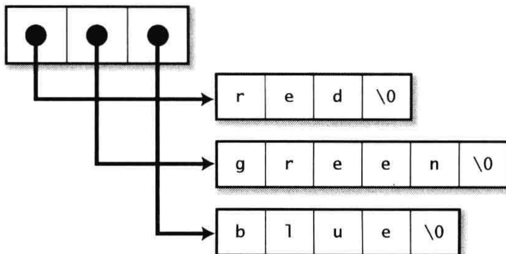
图 3-19 指针的数组
