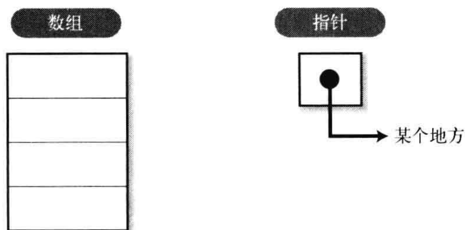
图 3-17 数组和指针
