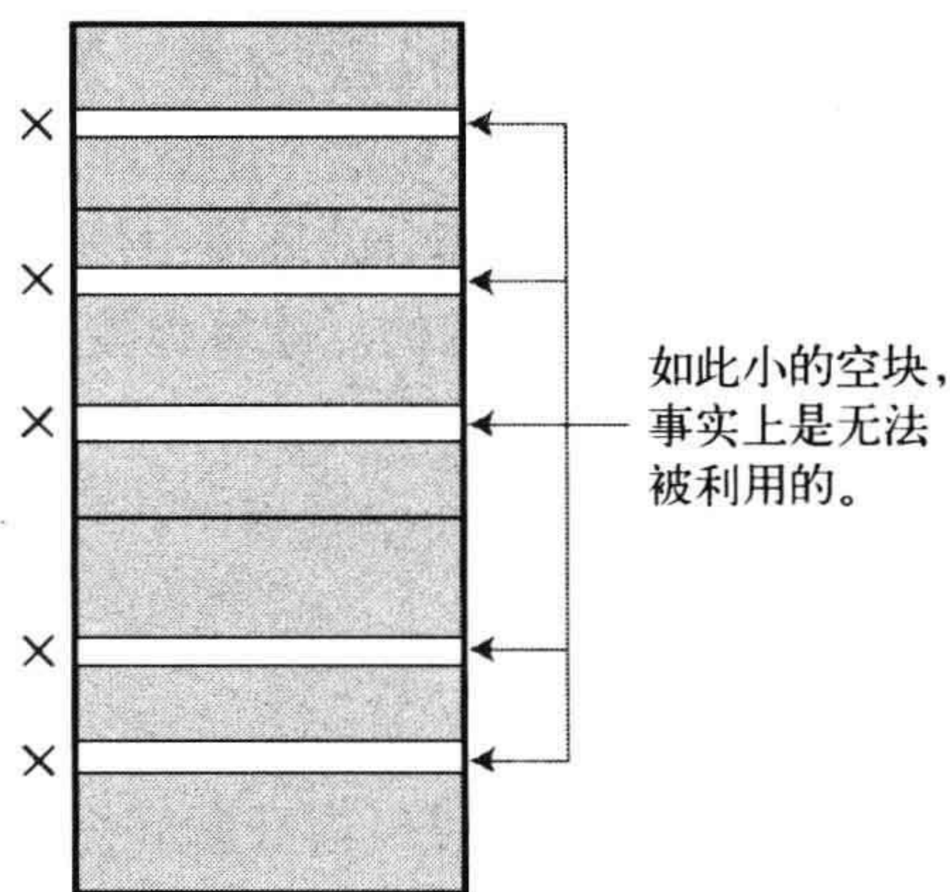
图 2-15 碎片化
