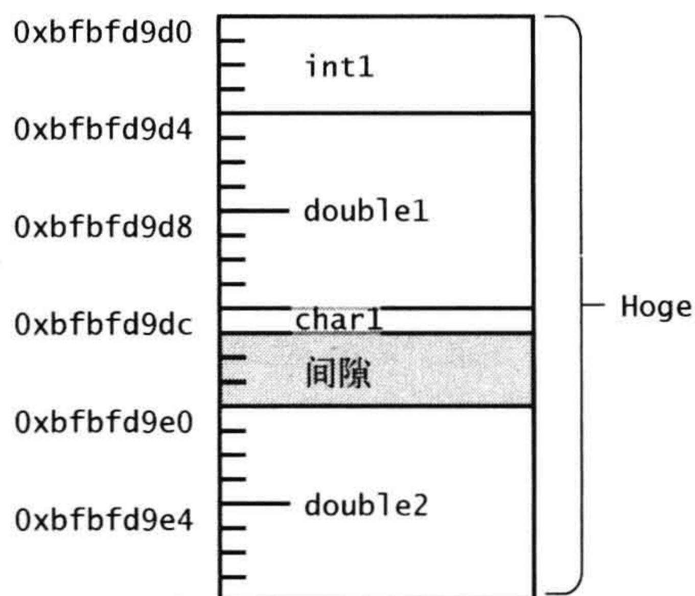
图 2-16 布局对齐
