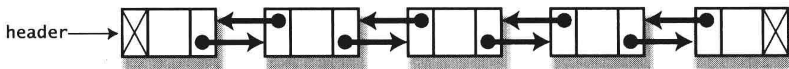
图 5-7 双向链表
